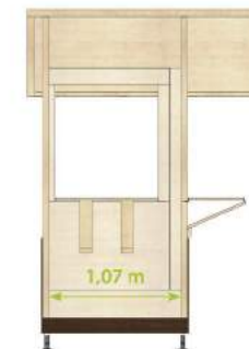
VISTA INTERNO LATO SINISTRO LINKE SEITENANSICHT INNEN INTERIOR VIEW LEFT SIDE
