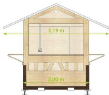
VISTA FRONTALE VORDERANSICHT FRONT VIEW
